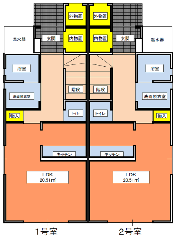
1階平面図
