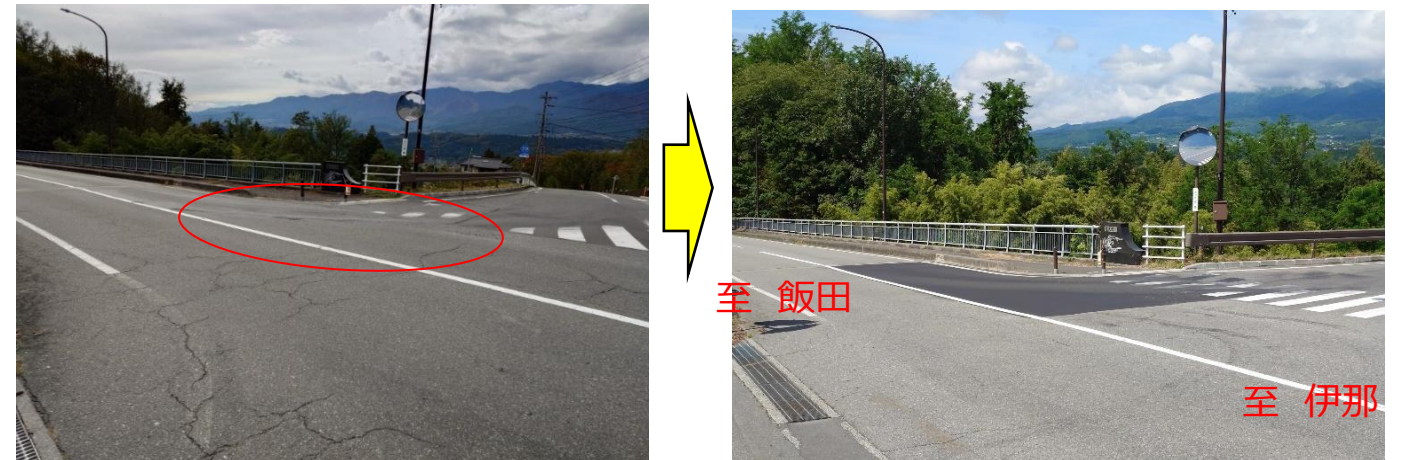
① 伊那生田飯田線 鳳来橋北交差点わだち (左: 対応前 右: JR対応済)
