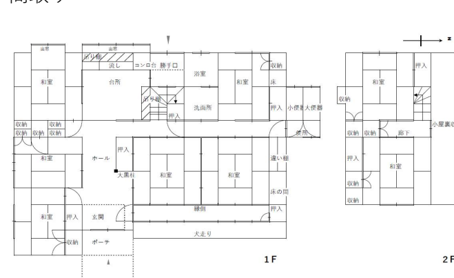
間取り
