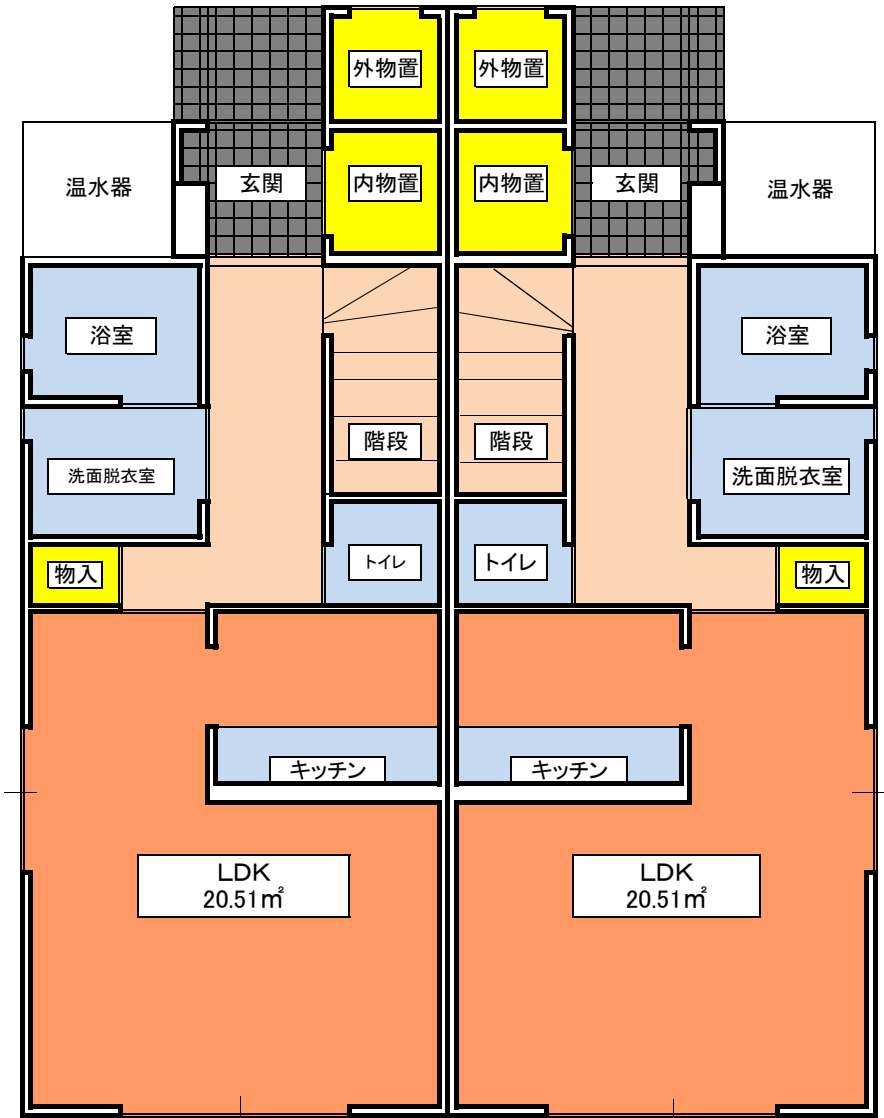
1階平面図
