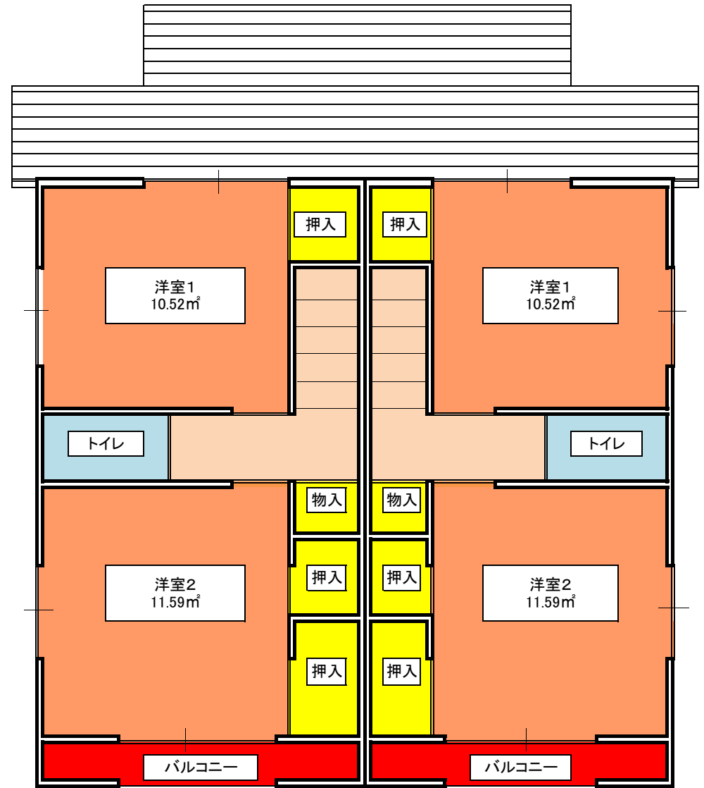
2階平面図
